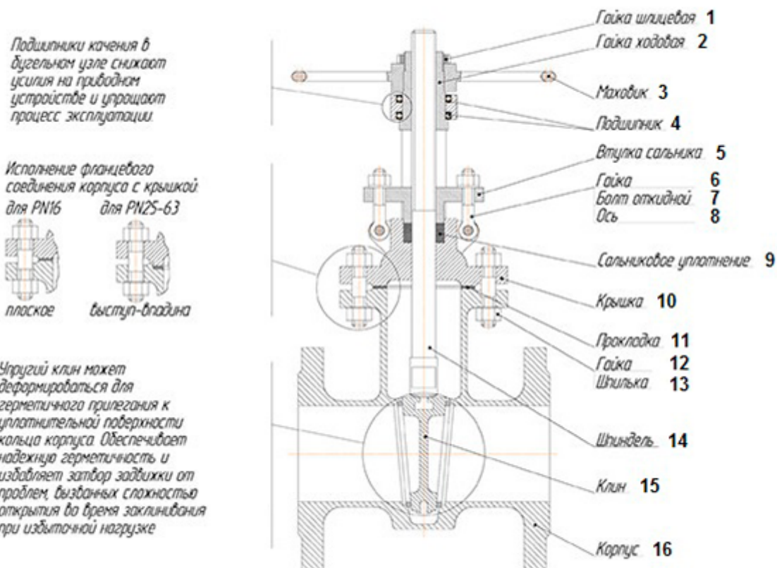
Структурная схема задвижек стальных клиновых 30с576нж с редуктором
