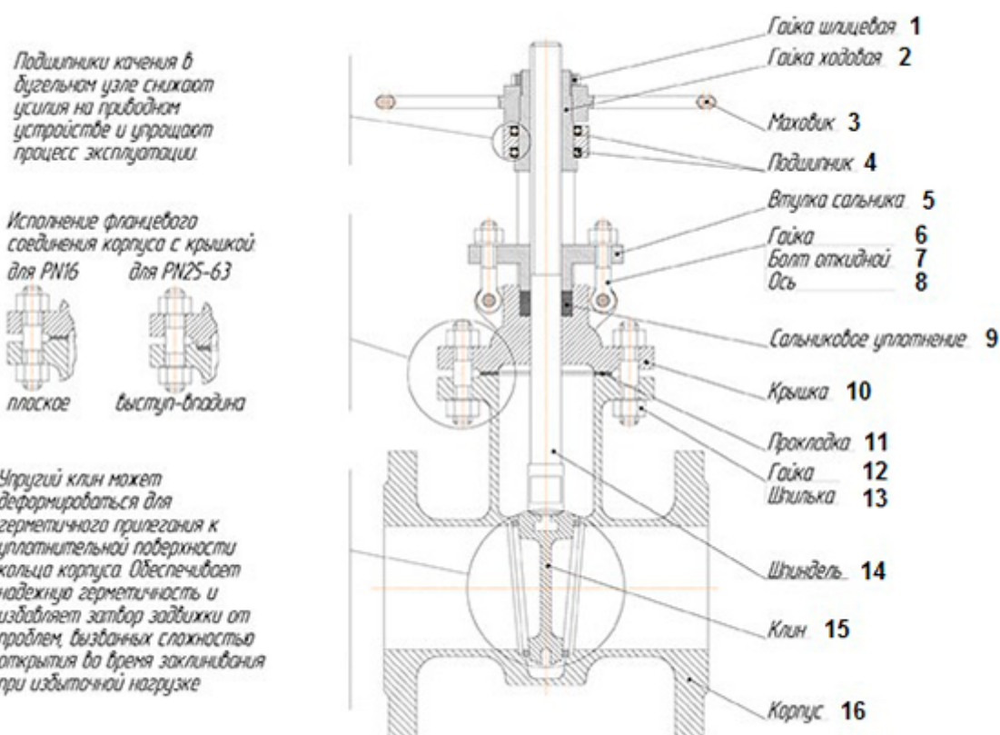
Структурная схема задвижек стальных клиновых 30нж599нж с редуктором
